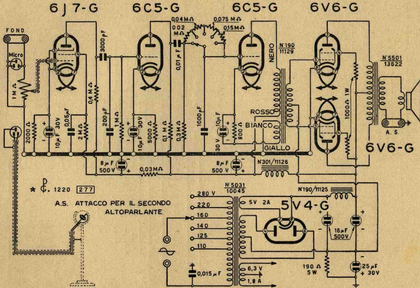
Lo schema elettrico dell'amplificatore G-5V.
